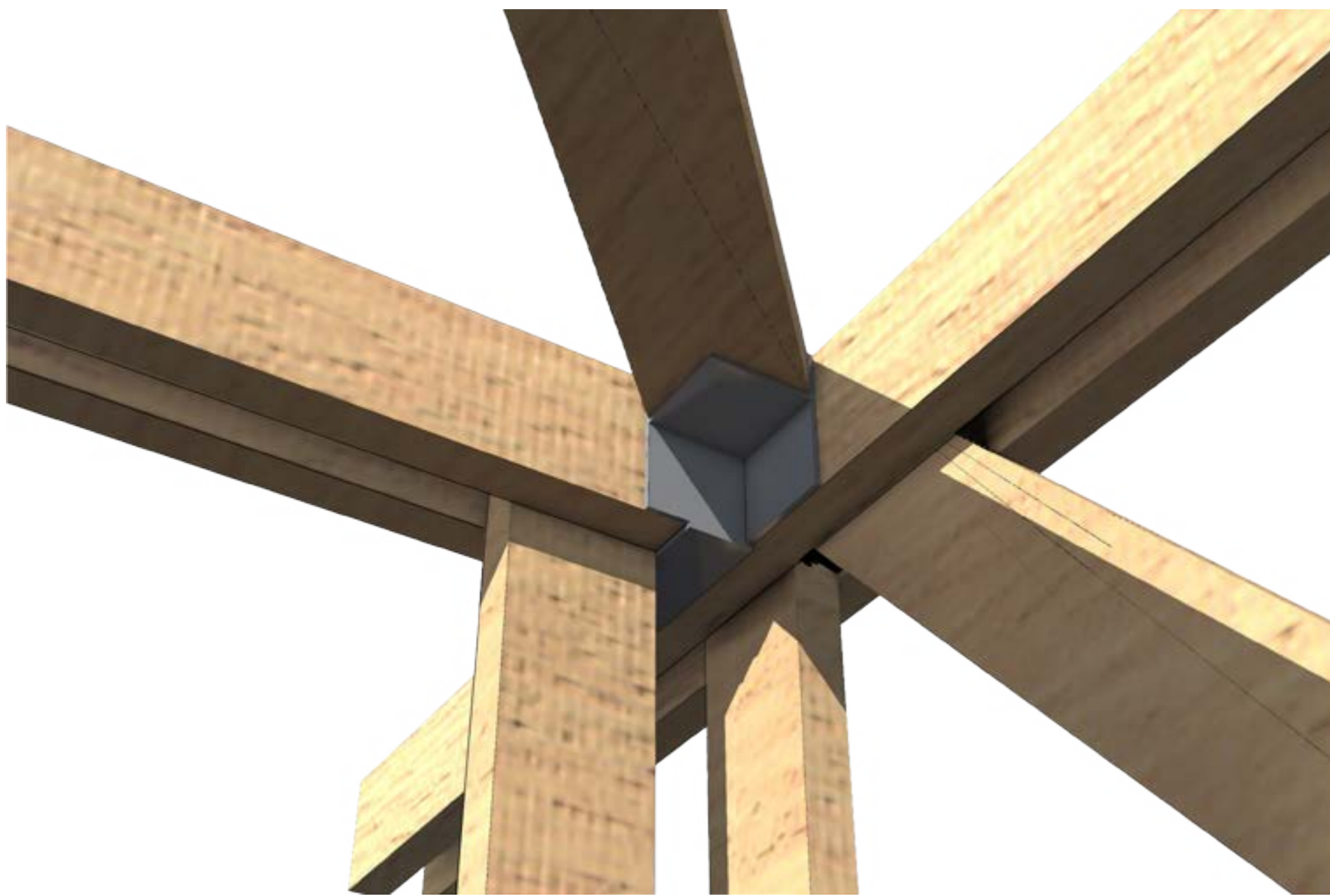
Détail d'assemblage
