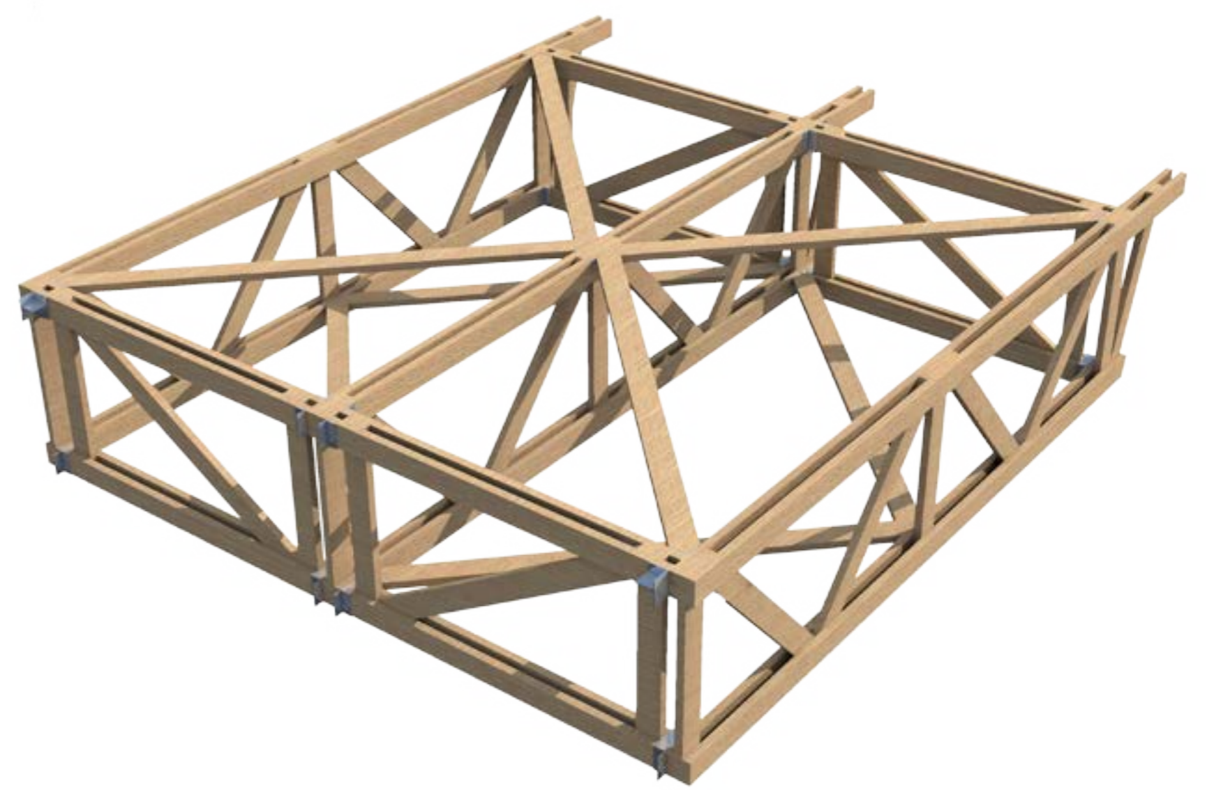
Triangulation de 2 demi-modules
