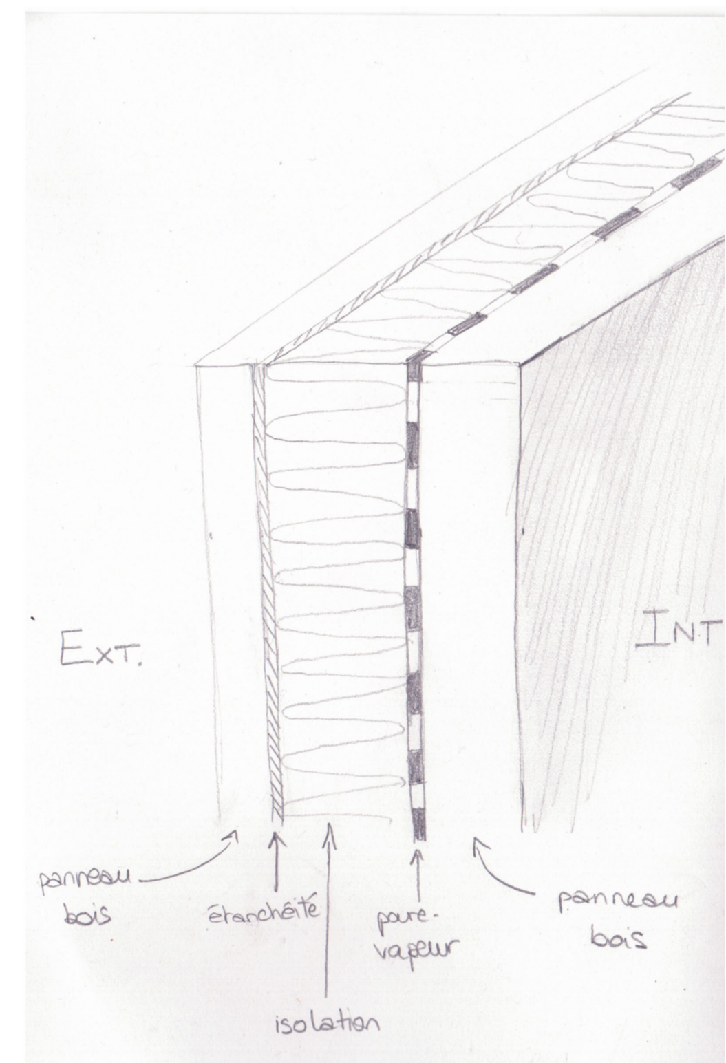
composition des panneaux de bois
