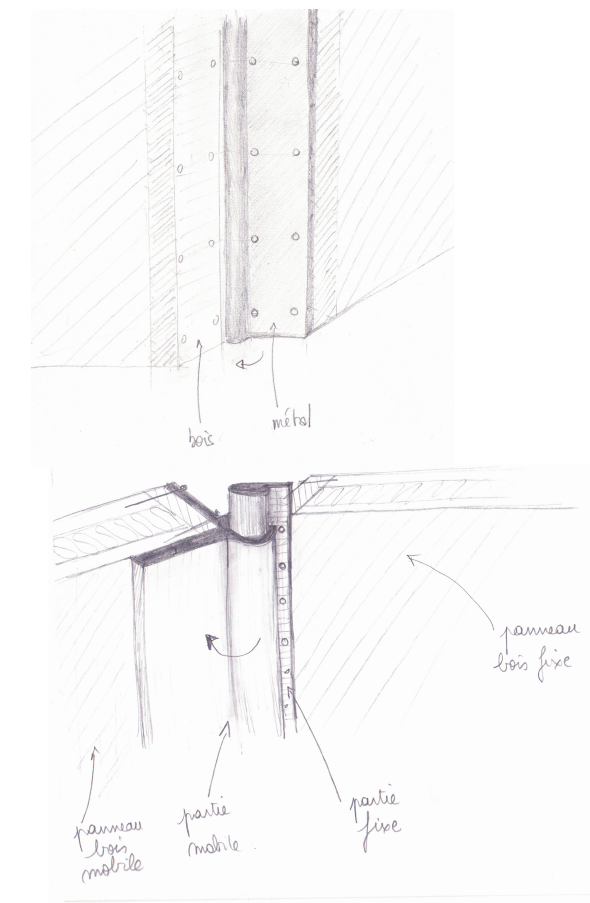
détails du pivot : axonométries
