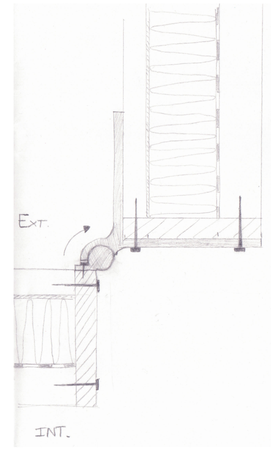
détails du pivot : plan
