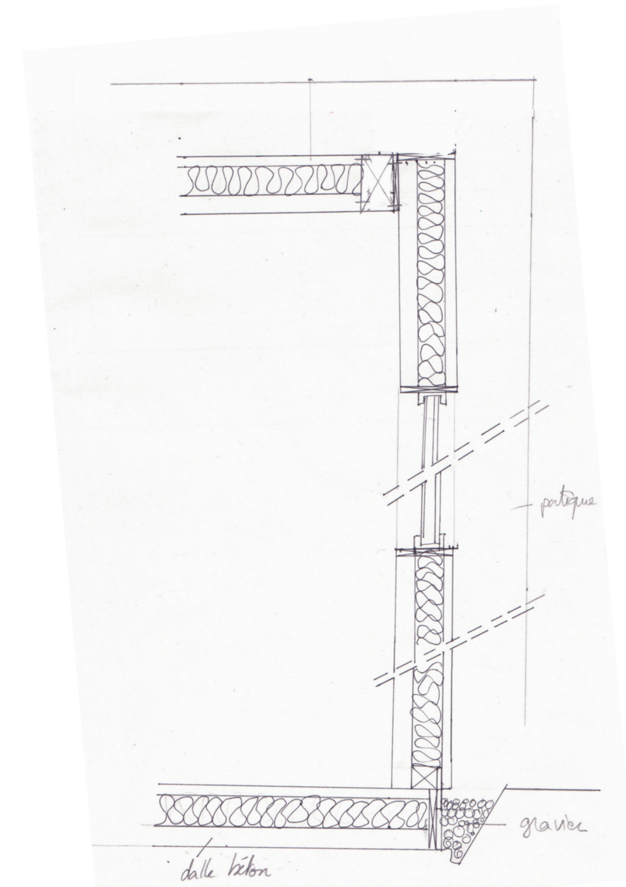
détail en au sol et en toiture
